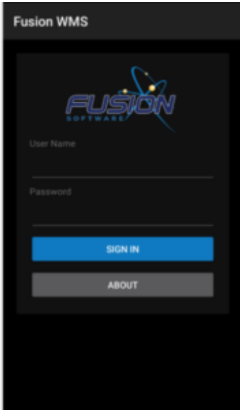
Login Page
